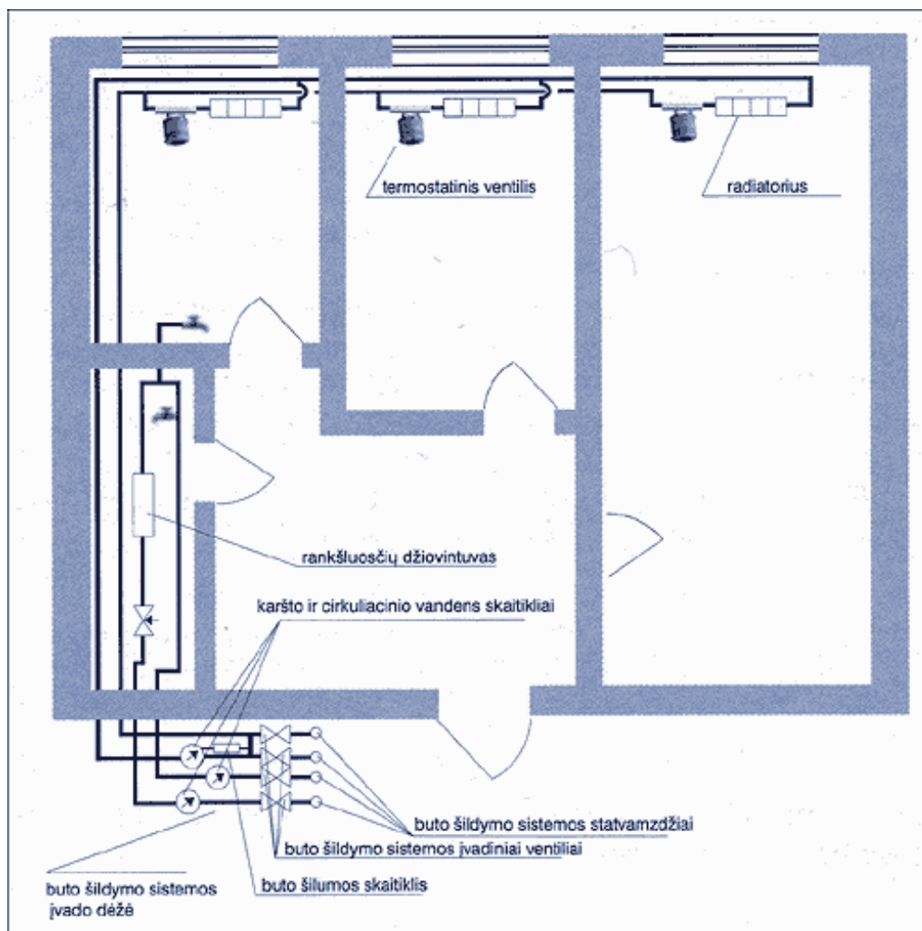
5 pav. Daugiabučio namo kolektovinė vieno buto šildymo ir karšto vandens tiekimo sistemos
